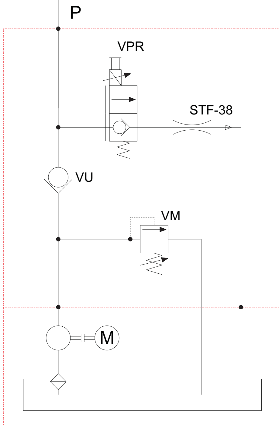
ESQUEMA HIDRÁULICO
